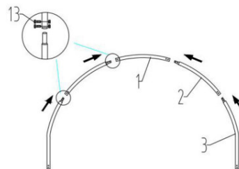
Zostavenie oblúka z jednotlivých rúr
