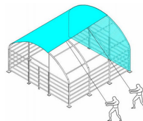
Preťahovanie strešnej plachty cez rám
