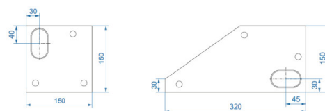
Pätky s otvormi na kotvy
