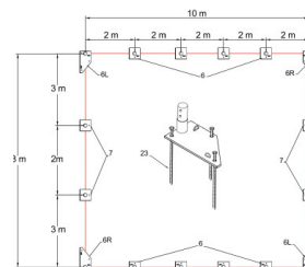
Príklad rozmiestnenia pätiiek (rozmery v m)
