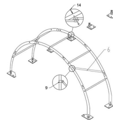
Diagonálne zavetrovanie
