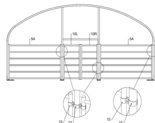
Rám prednej steny s dverami
