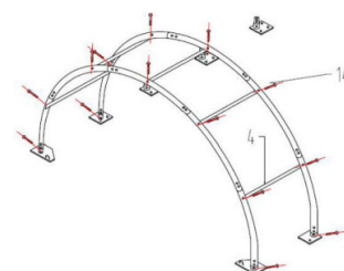
Spojenie oblúkov vážnicami
