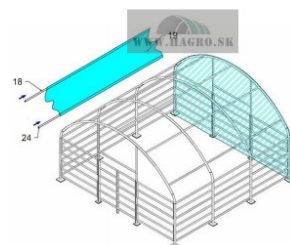
Napínacie rúry vo vreckách plachty
